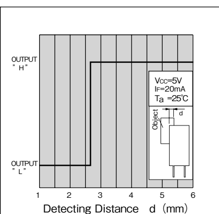
検出位置特性1(代表例) KI3531
