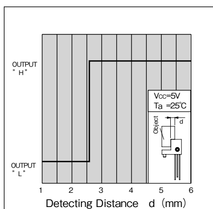
検出位置特性1(代表例) KI3731
